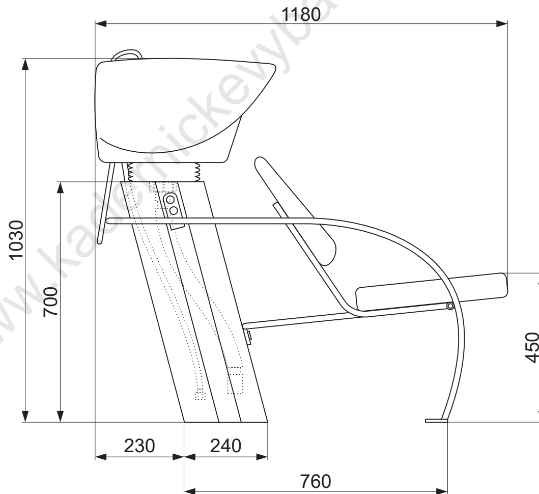
Boční pohled
