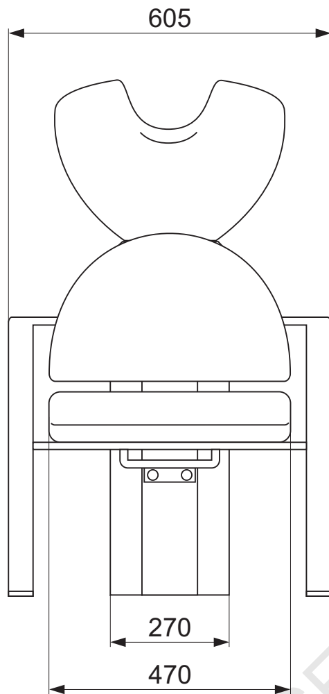
Čelní pohled
