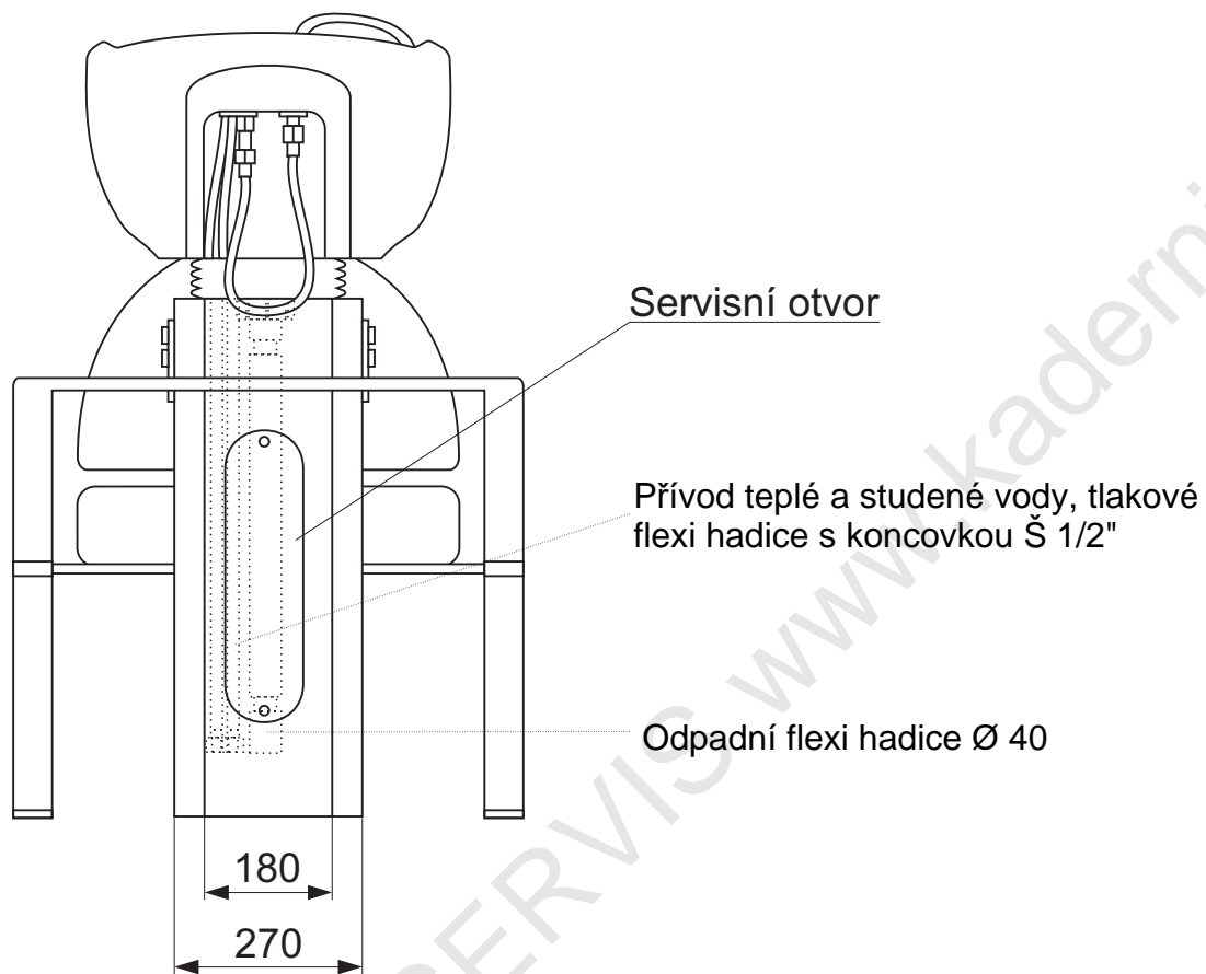
Zadní pohled
